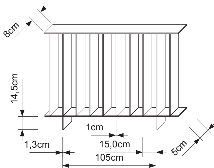
Bariera szczelinowa
