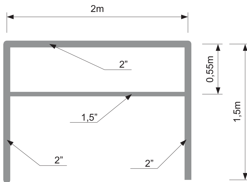
Bariera zabezpieczająca z pochwytym i przeciągiem moduł 2 m
