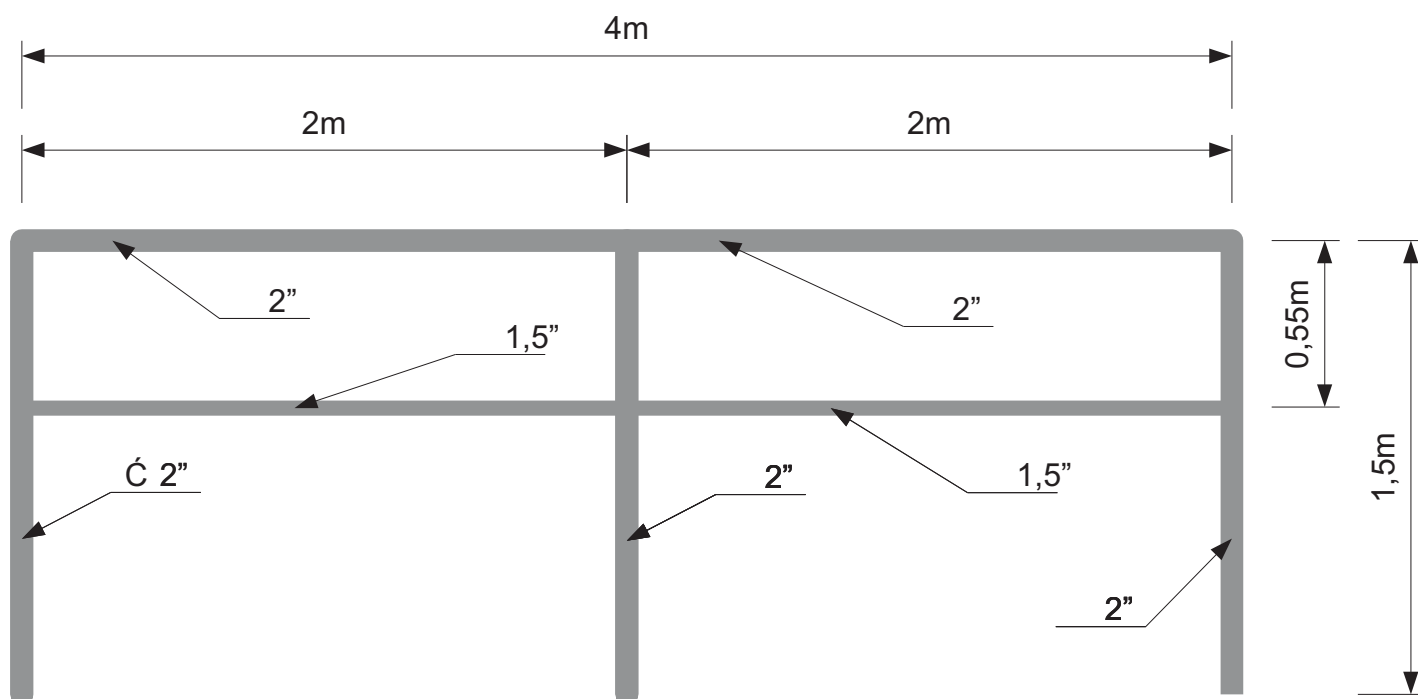
Bariera zabezpieczająca z pochwytym i przeciągiem moduł 4 m
