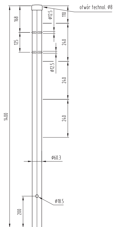
Słupek bariery zabezpieczającej „żółtej” moduł 2 m
