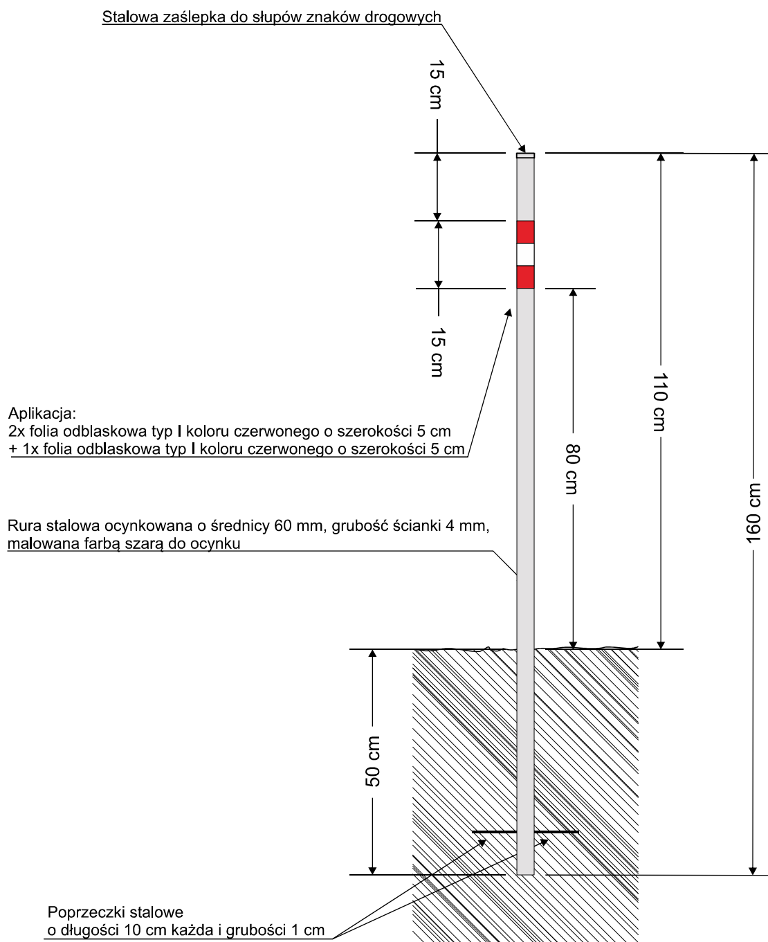
Słupek blokujący stalowy blokujący U-12c
